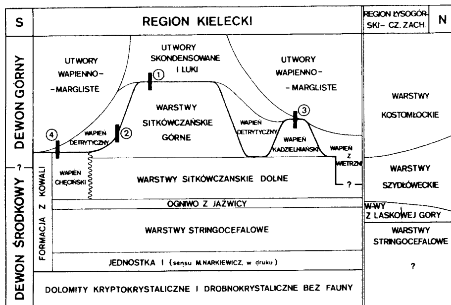
Fig. 2. Pozycja stratygraficzna i podział wewnętrzny formacji dolomitów i wapieni stromatoroidowo-koralowców z Kowali w regionie kieleckim i zachodniej części regionu łysogórskiego
