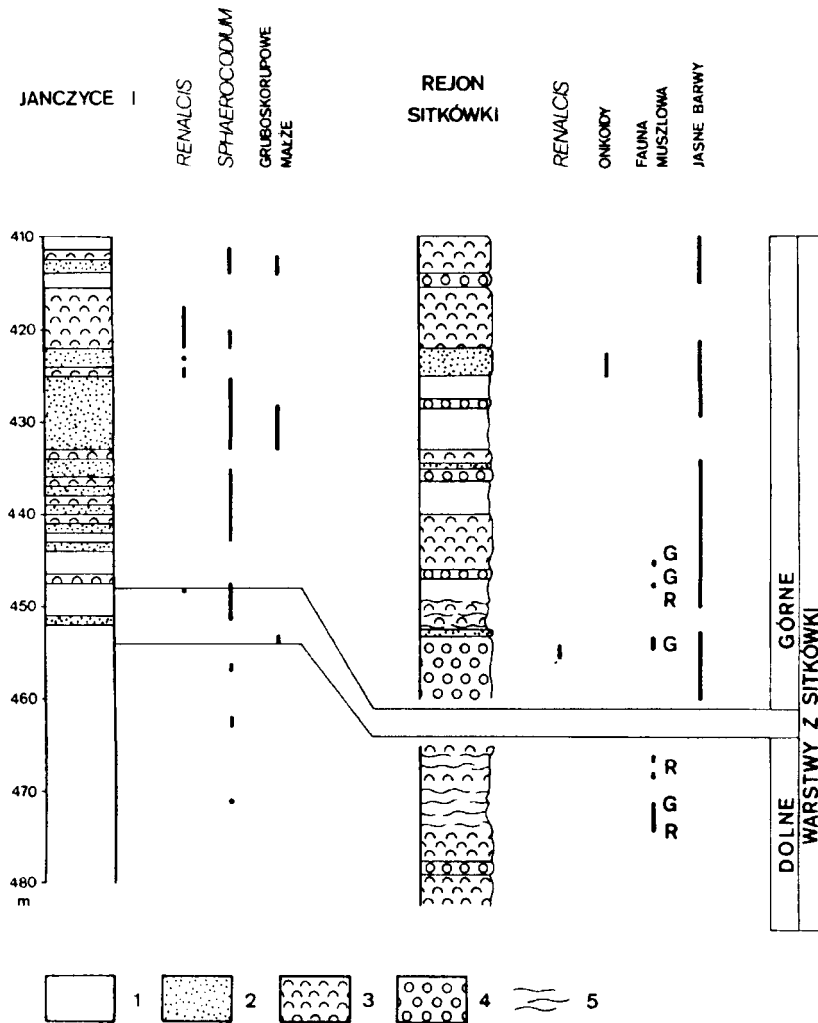
Fig. 4. Granica między dolnymi a górnymi warstwami z Sitkówki w profilach Janczyce I i w rejonie Sitkówki (ten ostatni według J. Kaźmierczaka, 1971b)
