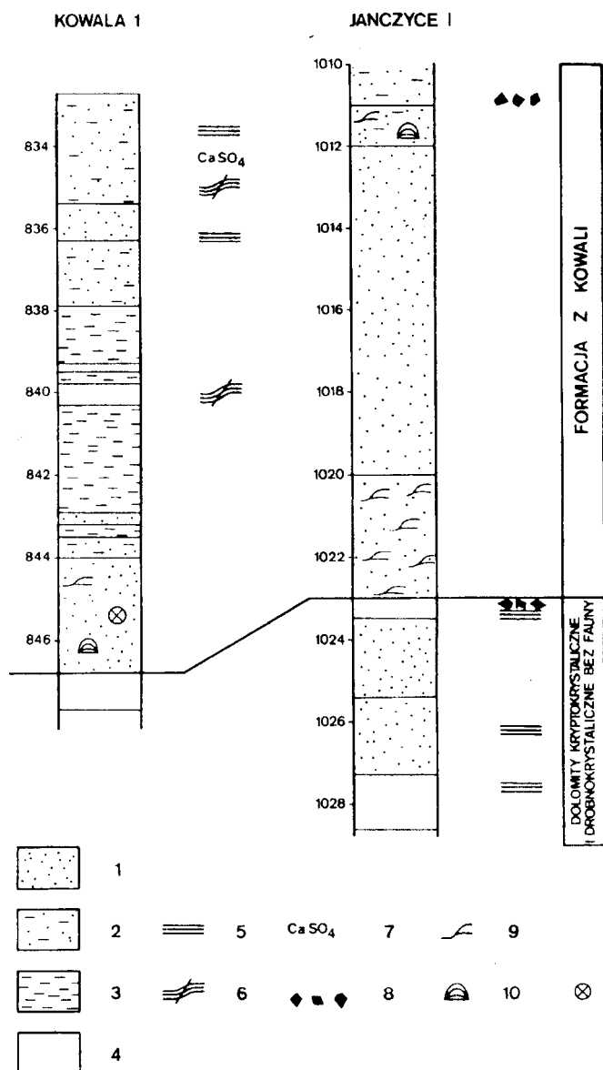
Fig. 3. Dolna granica formacji z Kowali w reperowych otworach wiertniczych Janczyce I i Kowala 1
